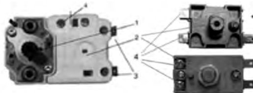
в) Модель Steatite (N3 CME, N4C (E)) г) модель O'Pro (S3S), EXPERT, TURBO, Steatite (S3C, S4CM, D400-2-BC, D325-2-BC)
